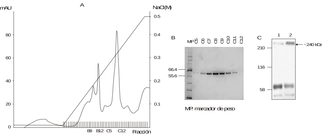
Figura 3. Obtención de la toxina CryAAC-R 423 S. A- Perfil cromatográfico de la purificación de CryAAC-R 423 S mediante FPLC; B- análisis de las fracciones del pico mayoritario mediante electroforesis SDS-PAGE al 12%. C- Ensayo de oligomerización: 1- CryAAC, 2- CryAAC-R 423 S.
